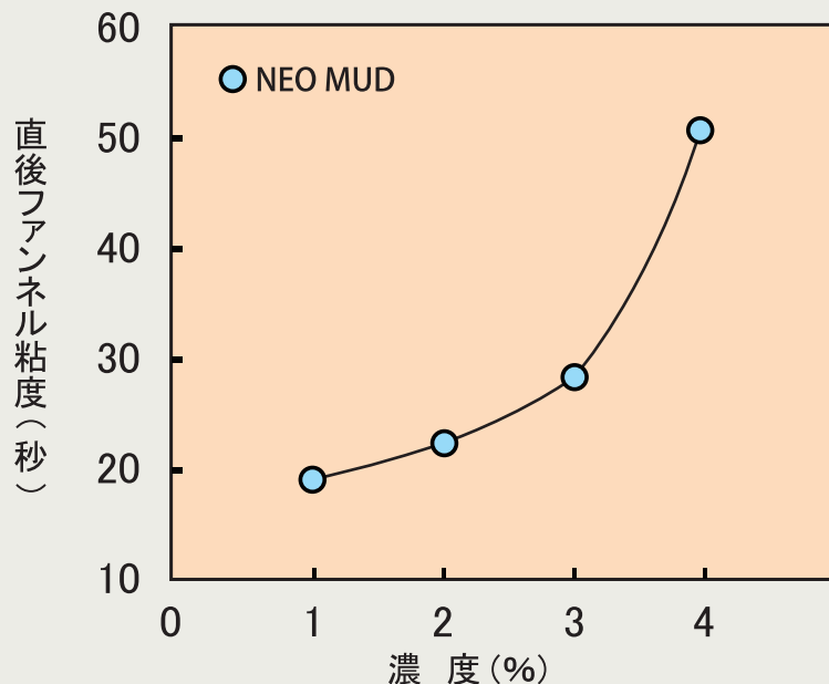
濃度とファンネル粘度の関係
