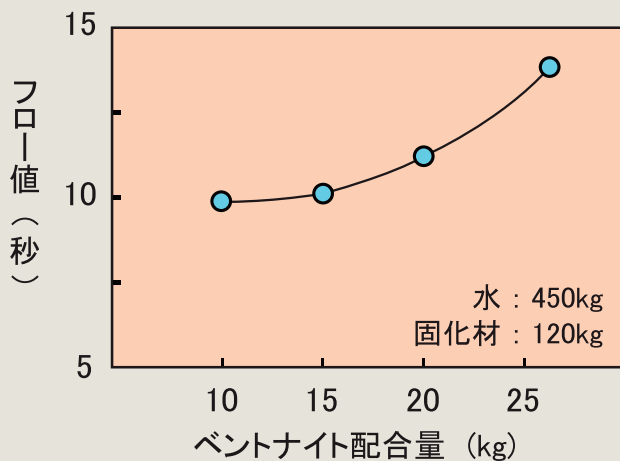
ベントナイト配合量と CB 粘性 (P フロー) の関係
