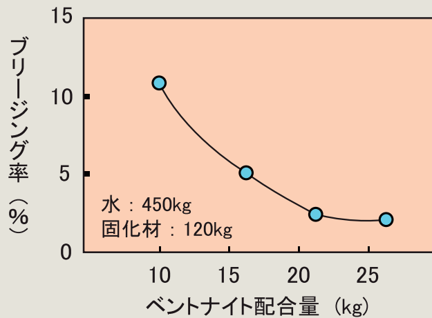
ベントナイト配合量と CB ブリージング率の関係
